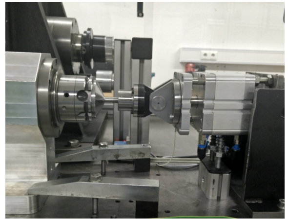
Bild 2: Belastungsprüfstand
