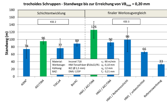
Bild 2: Standwege beim trochoiden Schruppfräsen: links Schichtentwicklung; rechts Werkzeugvergleich
